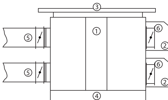
Rys. 17. Akcesoria zewnętrzne
