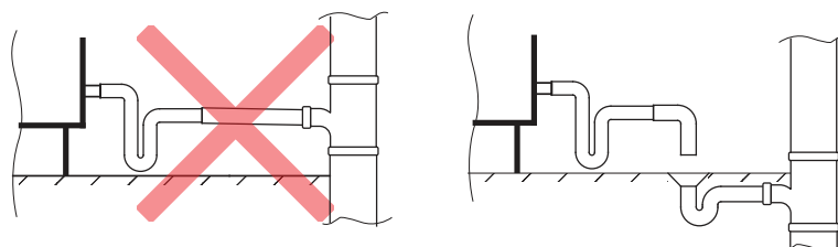
Rys. 16. Podłączenie odpływu skroplin do kanalizacji
