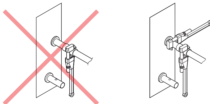
Rys. 12. Podłączanie tulei
