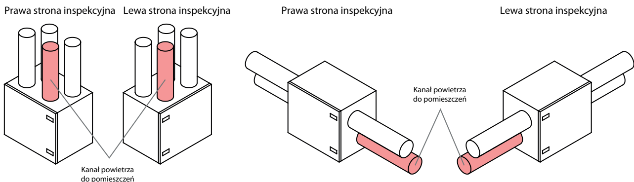
Rys. 3. Klasyfikacja central według stron inspekcyjnych
