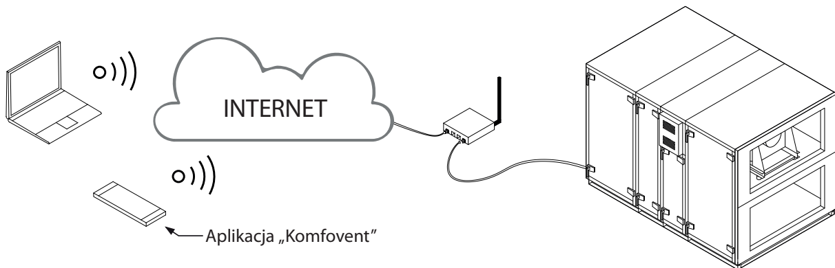
Rys. 28. Przykłady połączenia centrali z Internetem lub siecią lokalną
