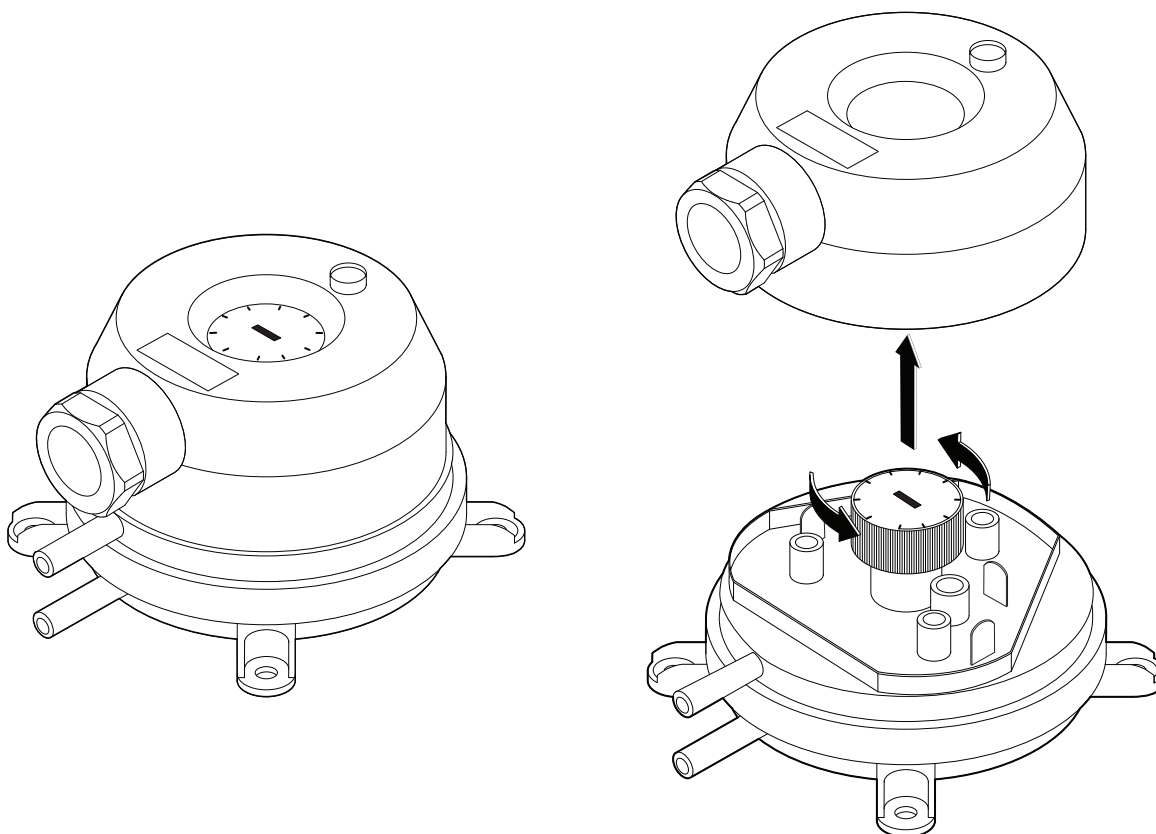
Rys. 29. Przelącznik ciśnieniowy
