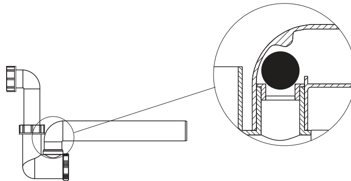
Rys. 15. Przykład syfonu z zaworem jednokierunkowym
