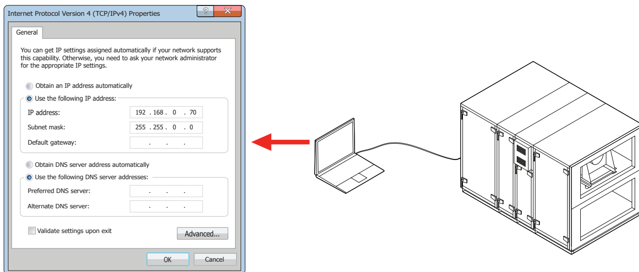
Rys. 27. Ustawienia sieci komputerowej do bezpośredniego połączenia z centralą
