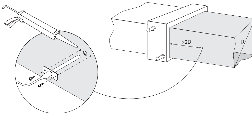
Rys. 22. Montaż czujnika temperatury powietrza nawiewanego
