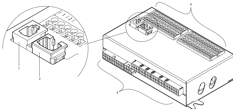
Rys. 18. Płyta główna C5
