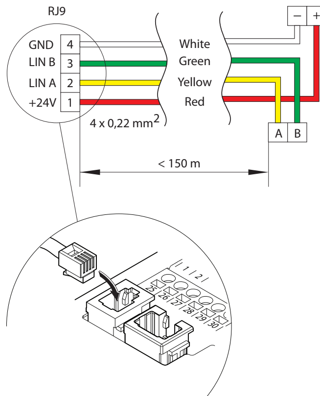
Rys. 23. Schemat podłączenia panelu sterowniczego
