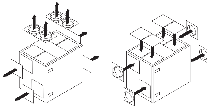
Rys. 2. Przeniesienie króćców przyłączeniowych kanałów central uniwersalnych
