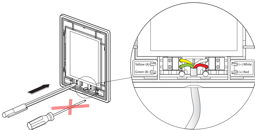
Rys. 24. Schemat podłączenia panelu sterowniczego
