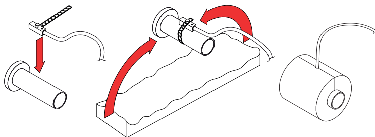
Rys. 13. Montaż czujnika temperatury wody powrotnej
