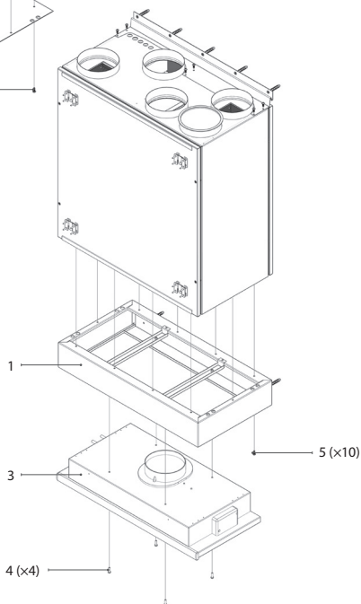
Rys. 12c. Montaż okapu kuchennego 392-12
