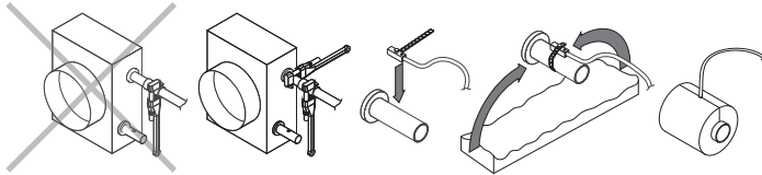
Rys. 16. Podłączanie przewodów nagrzewnicy/chłodziцы wodnej i instalowanie czujnika temperatury wody powrotnej
