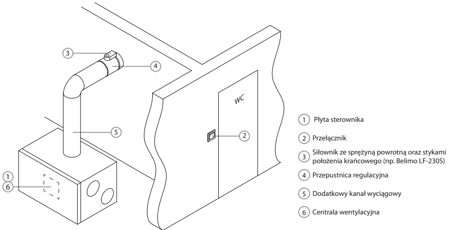
Rys. 9. Przykład montażu dodatkowego kanału wyciągowego
