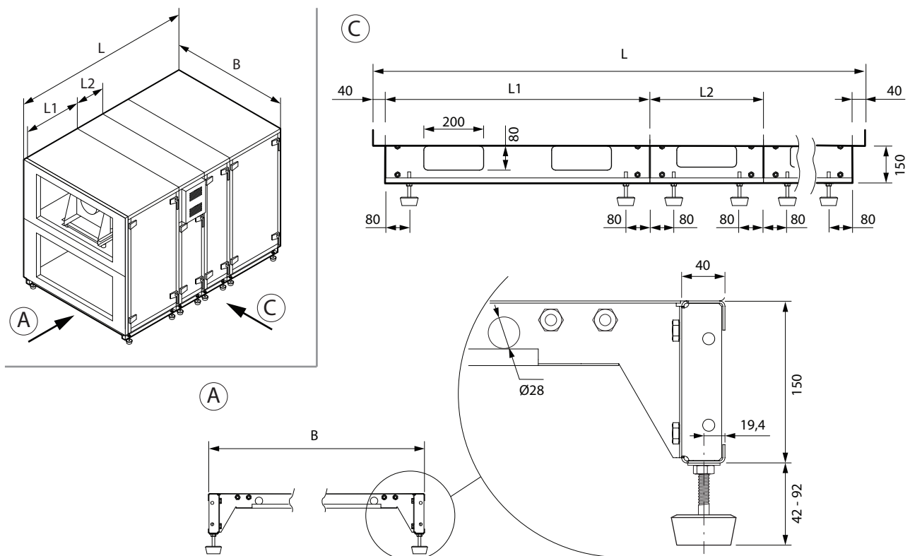
Rys. 17. Rama montażowa z regulowanymi nóżkami
