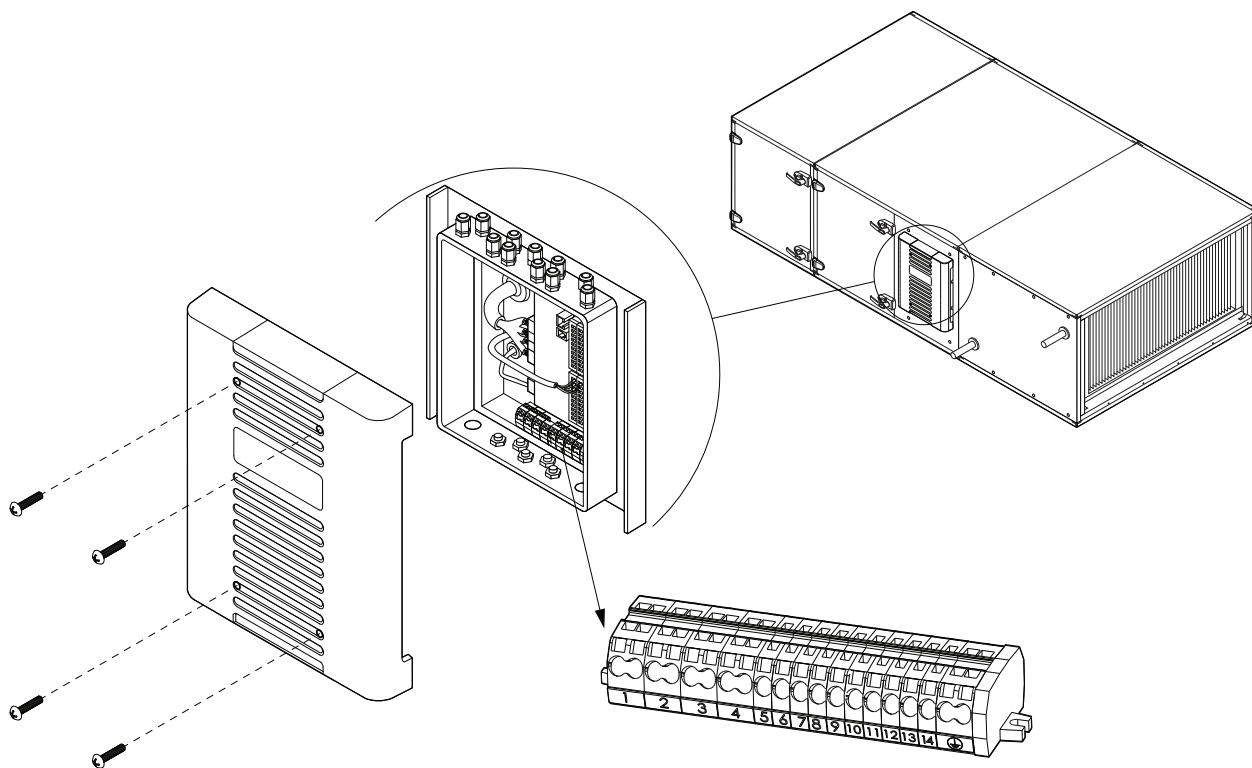
Rys. 45. Zaciski przyłączeniowe central wentylacyjnych VERSO RA
