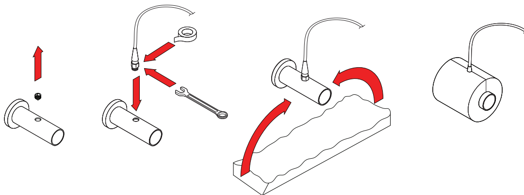
Rys. 27. Montaż czujnika temperatury wody powrotnej z gwintem 1
