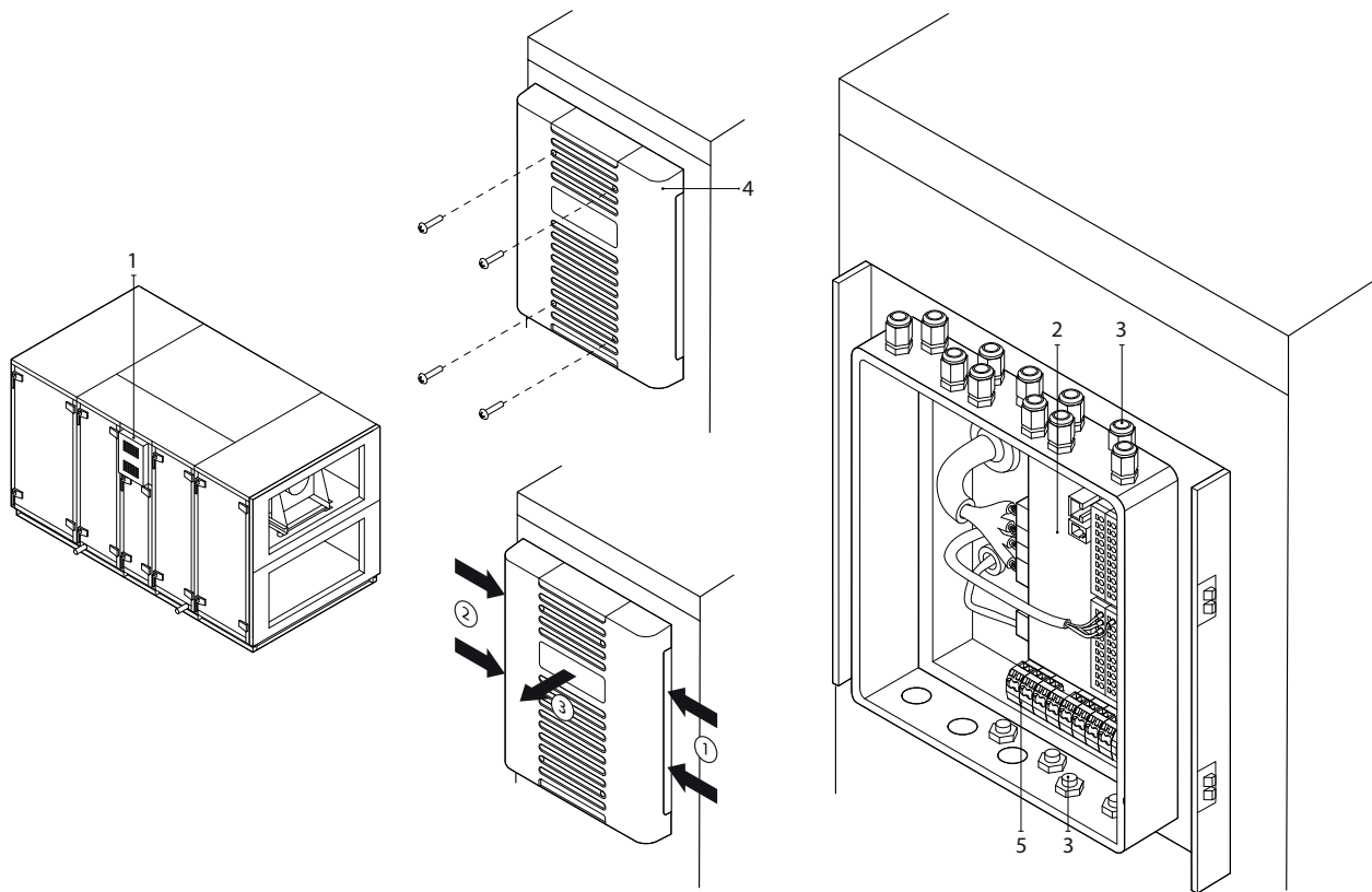
Rys. 36. Skrzynka automatyki
