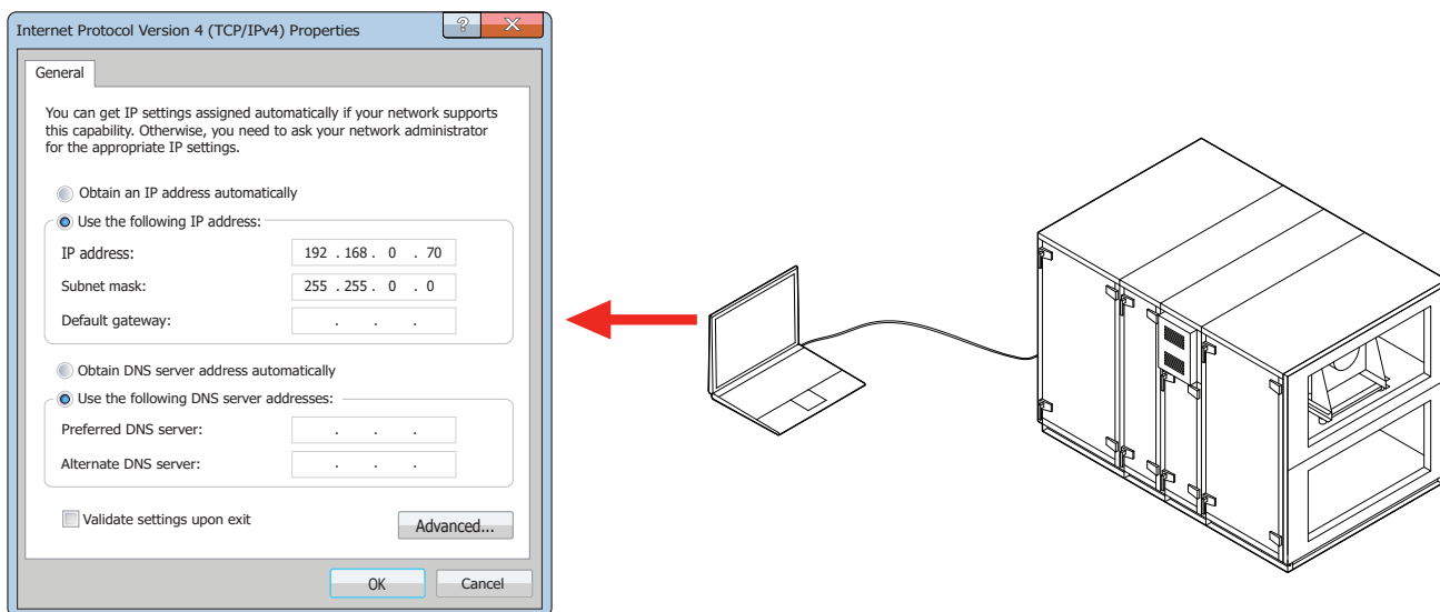
Rys. 52. Ustawienia sieci komputerowej do bezpośredniego połączenia z centralą
