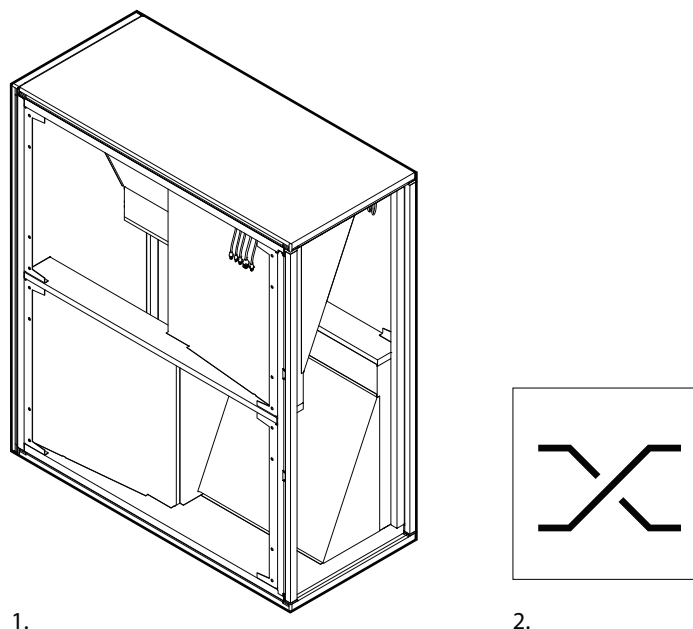
Rys. 12. Sekcja zmiany kierunku przepływu powietrza 1 – sekcja zmiany przepływu powietrza, 2 – tabliczka sekcji
