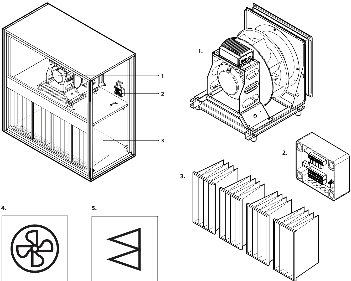
Rys. 1. Sekcja filtr-wentylator
