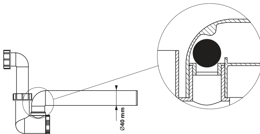
Rys. 29. Przykład syfonu z zaworem jednokierunkowym
