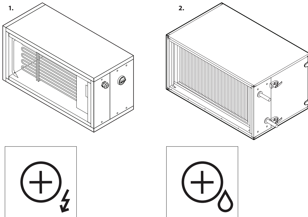
Rys. 7. Sekcja nagrzewnicy
