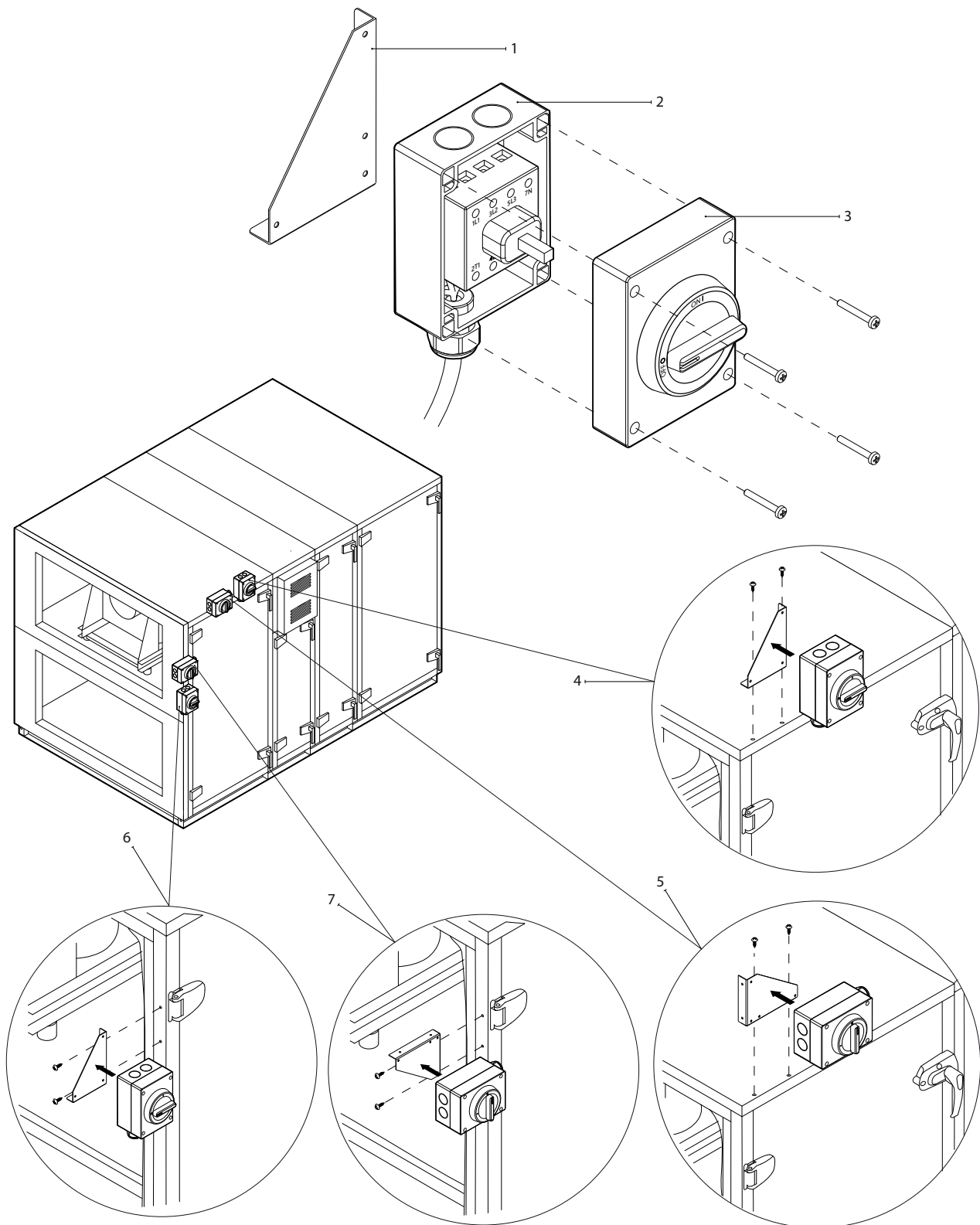
Rys. 34. Wyłącznik główny i przykłady jego montażu
