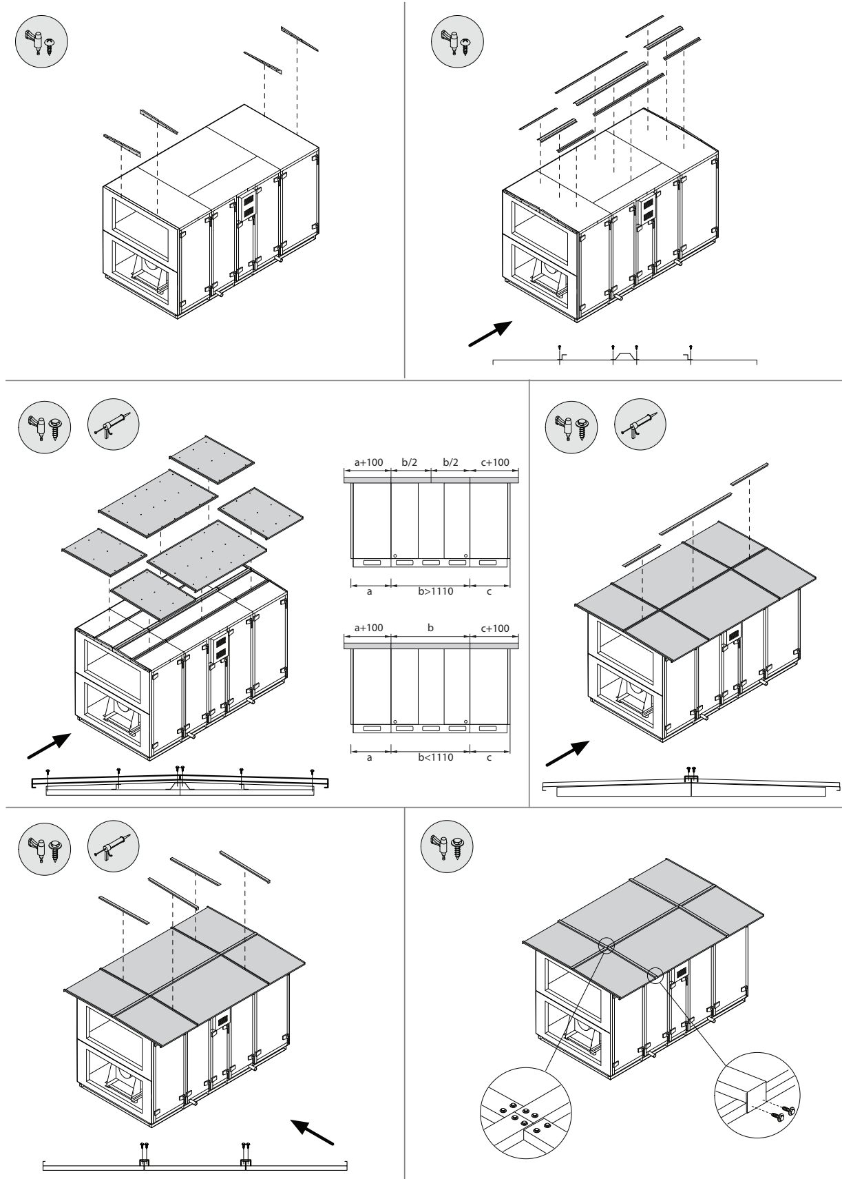
Rys. 33. Montaż osobno zamawianego dachu ochronnego 1
