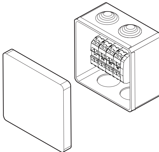
Rys. 50. Skrzynka przyłączeniowa PD1
