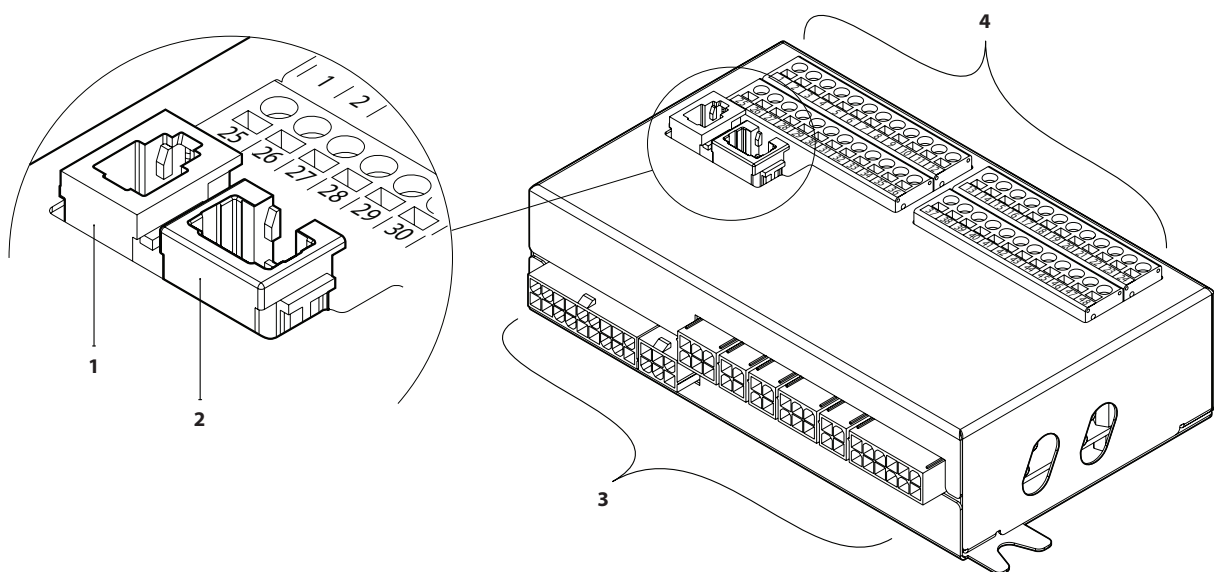
Rys. 37. Płyta główna panelu sterowniczego C5
