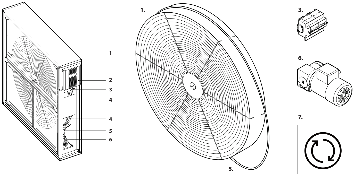
Rys. 3. Sekcja rekuperatora obrotowego
