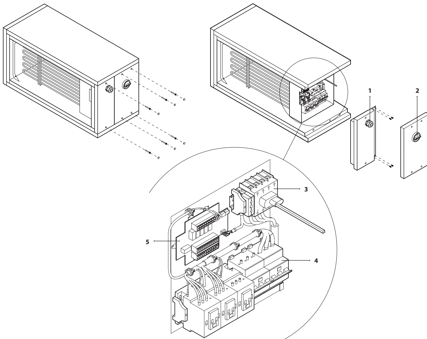
Rys. 35. Wyłącznik główny wewnątrz sekcji nagrzewnicy elektrycznej 1 – przelotka kabla doprowadzającego, 2 – uchwyt pokrętła głównego wyłącznika, 3 – wyłącznik główny, 4 – przełącznik automatyczny, 5 – elektroniczna płytką drukowaną sterowania nagrzewnicą
