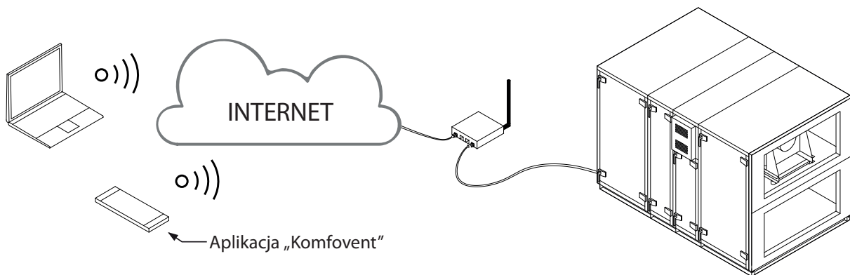
Rys. 53. Przykłady połączenia centrali z Internetem lub siecią lokalną
