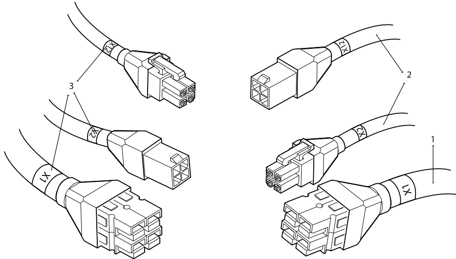
Rys. 49. Połączenia kablowe między sekcjami
