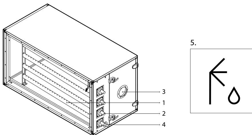
Rys. 10. Sekcja nawilżacza
