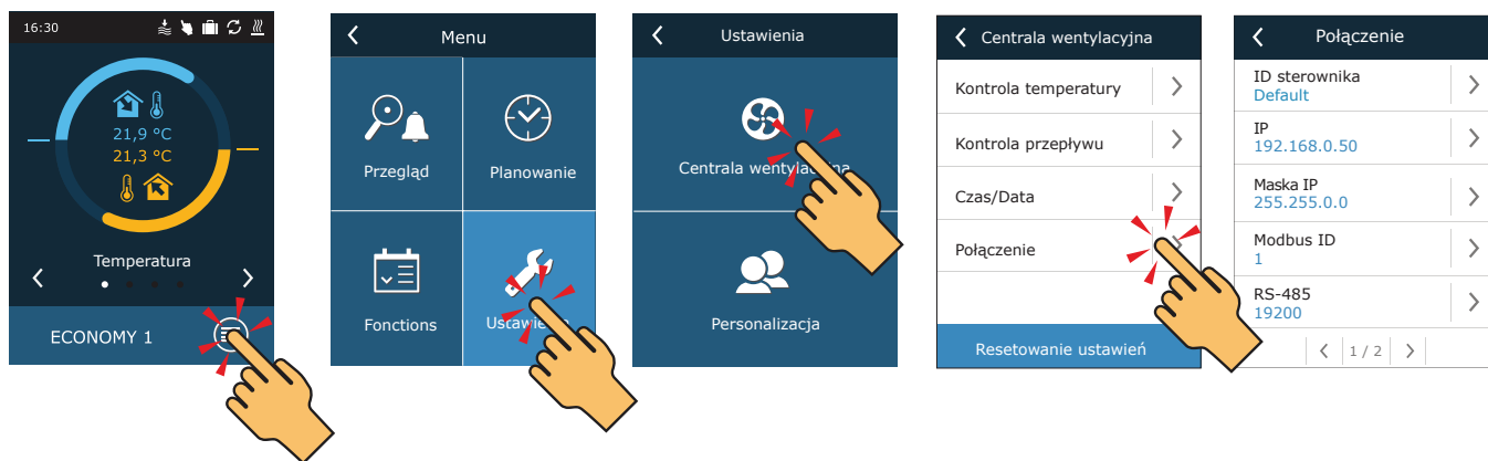
Rys. 51. Adres IP można zobaczyć i zmienić na panelu sterowniczym
