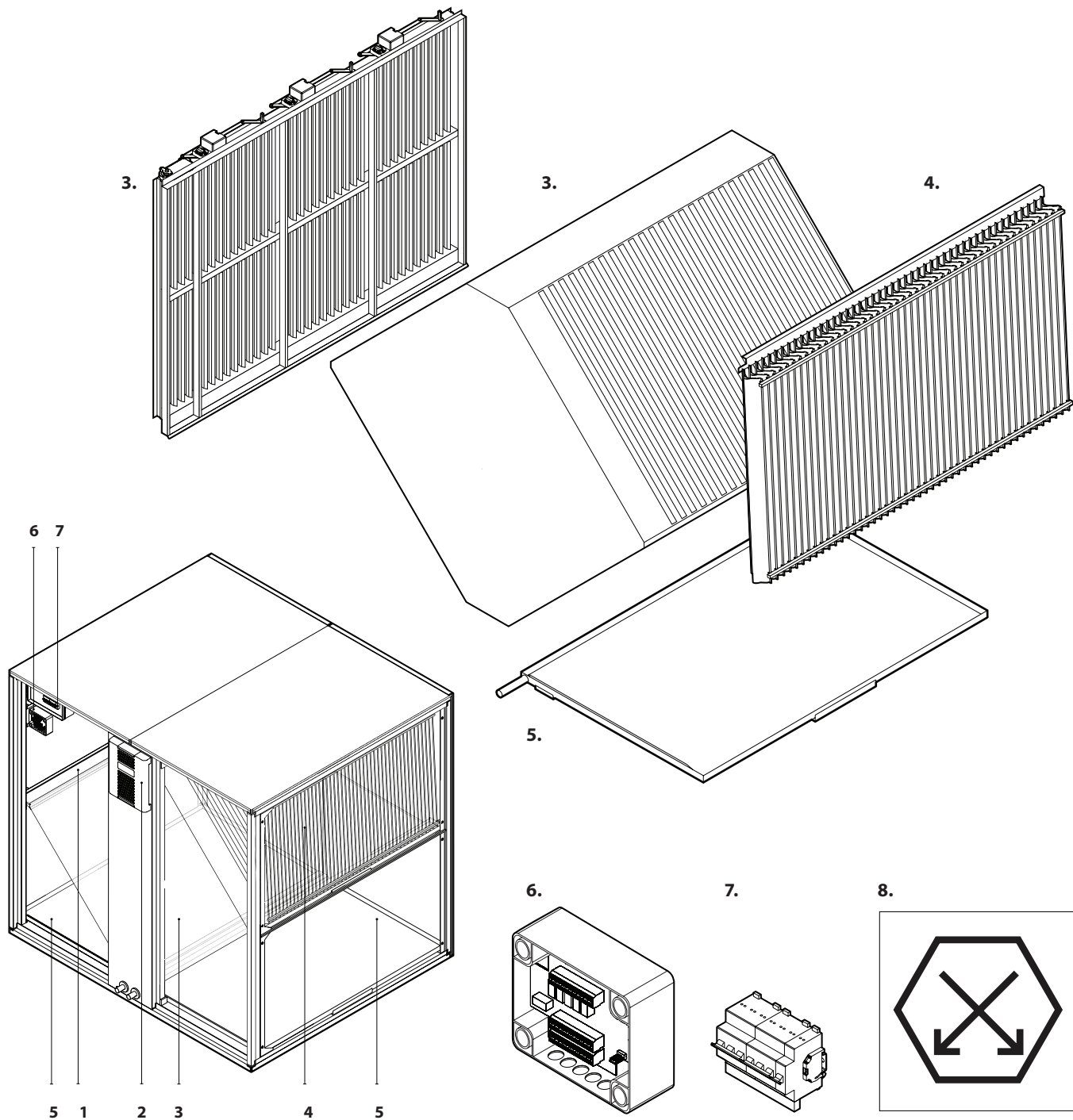
Rys. 2. Sekcja przeciwprądowego wymiennika ciepła (CF)
