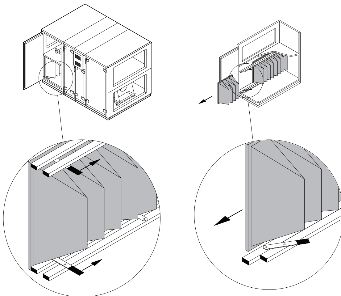
Rys. 54. Urządzenie mocujące filtr
