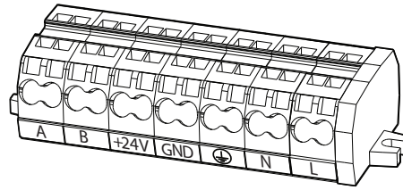
Rys. 43. Dodatkowa listwa zaciskowa
