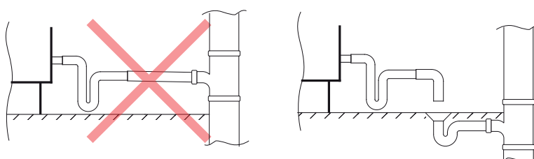
Rys. 30. Przyłącze spustu kondensatu do instalacji kanalizacyjnej
