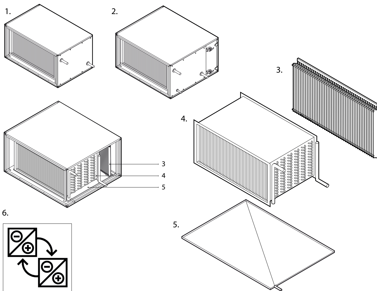
Rys. 4. Sekcje wymiennika ciepła z cieczą pośredniczącą
