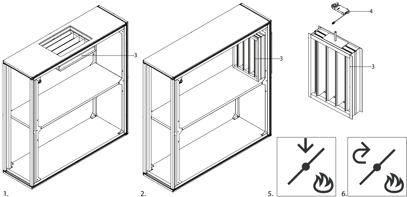
Rys. 11. Sekcja oddymiania
