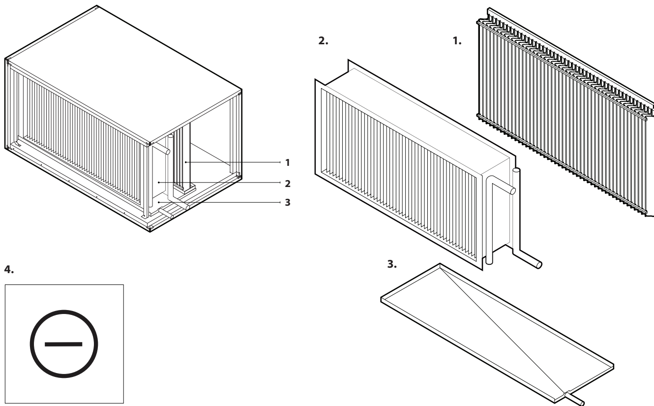
Rys. 5. Sekcja chłodnicy
