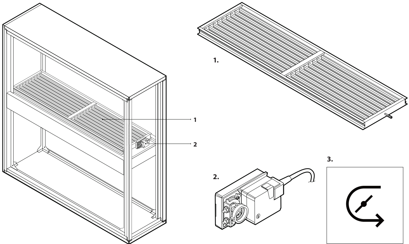
Rys. 4. Sekcja recyrkulacji
