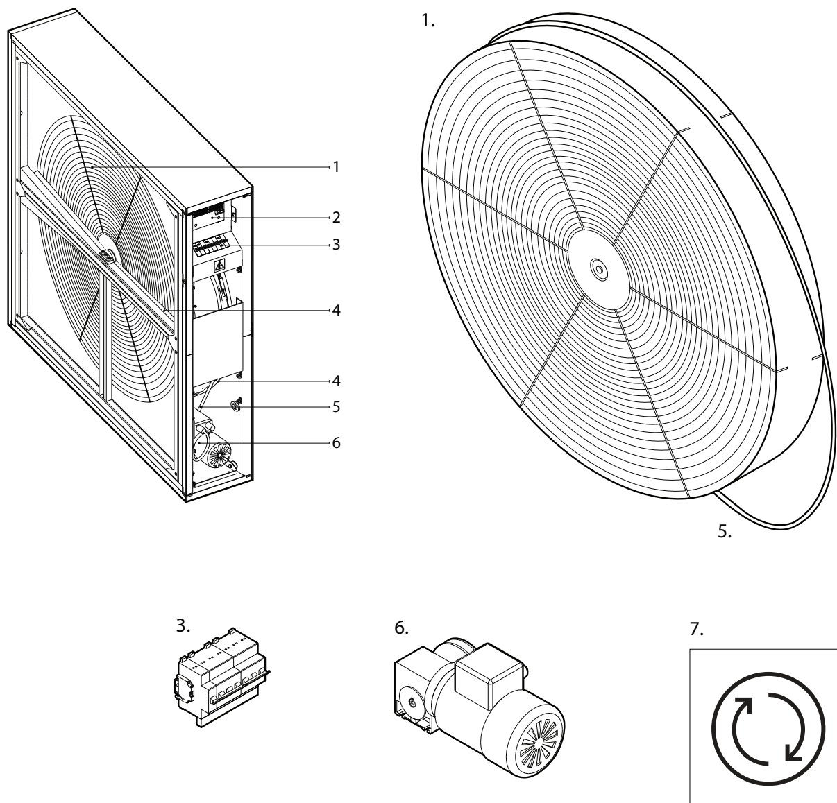
Rys. 3. Sekcja rekuperatora obrotowego
