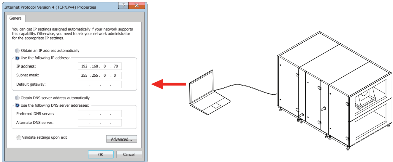
Rys. 42. Ustawienia sieci komputerowej do bezpośredniego połączenia z centralą
