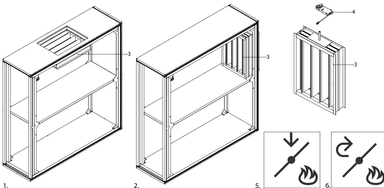
Rys. 9. Sekcja oddymiania
