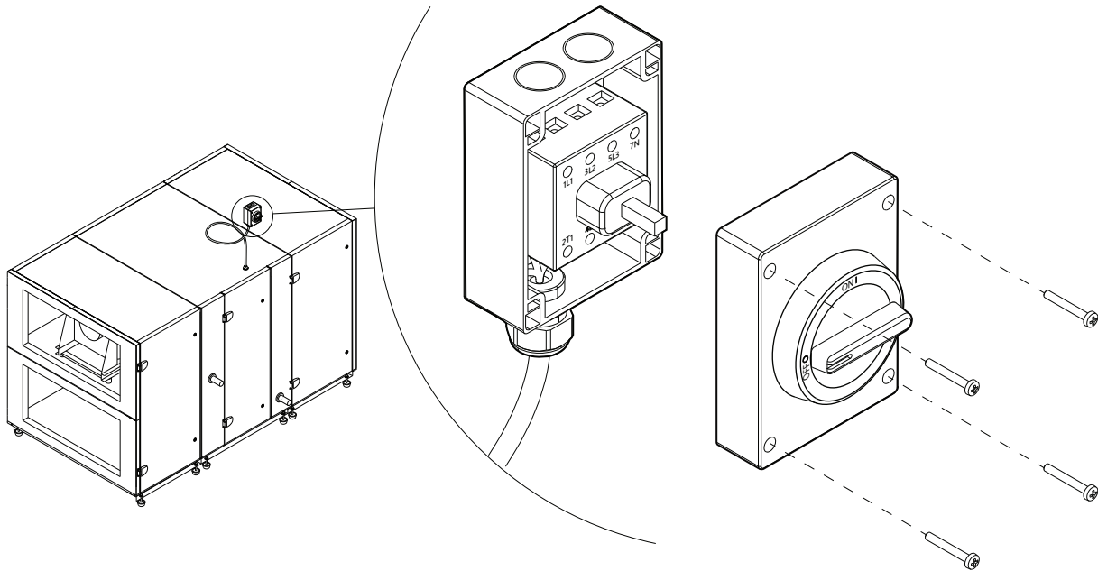
Rys. 28. Wyłącznik główny
