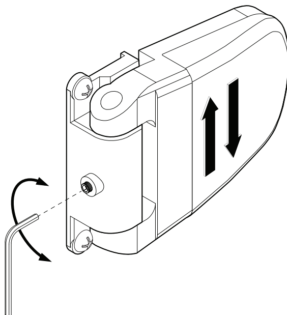
Rys. 14. Regulacja zawiasów
