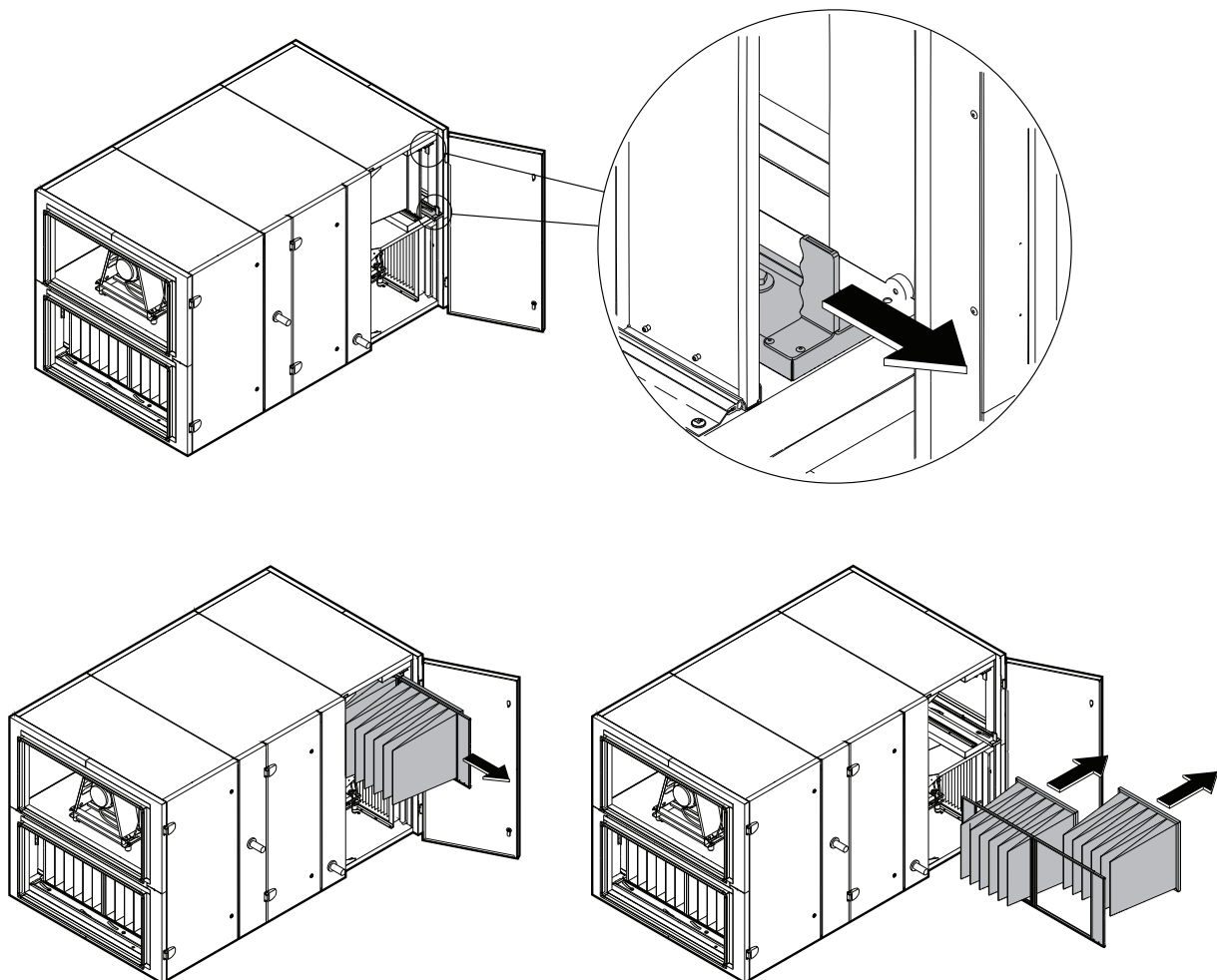
Rys. 44. Urządzenie mocujące filtr
