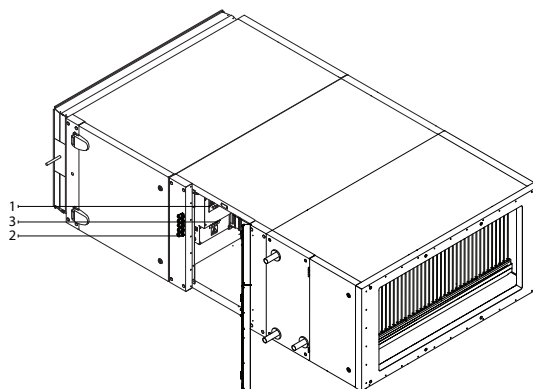
Rys. 30. Skrzynka automatyki
