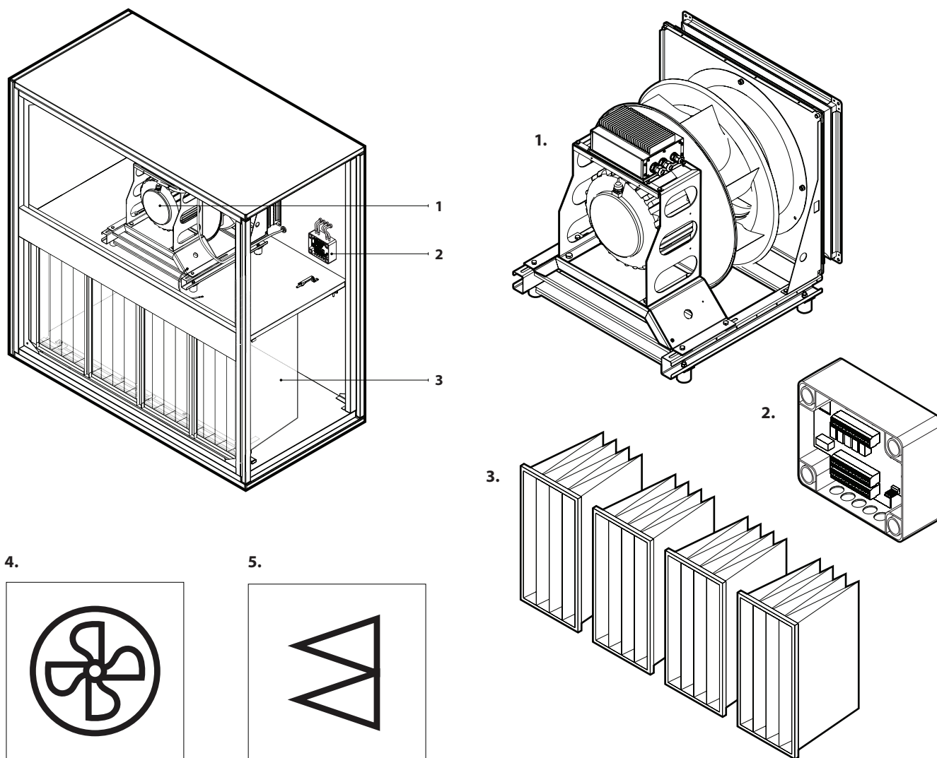
Rys. 1. Sekcja filtr-wentylator
