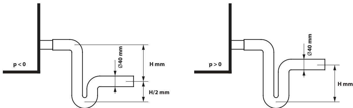
Rys. 21. Montaż syfonu bez zaworu jednokierunkowego
