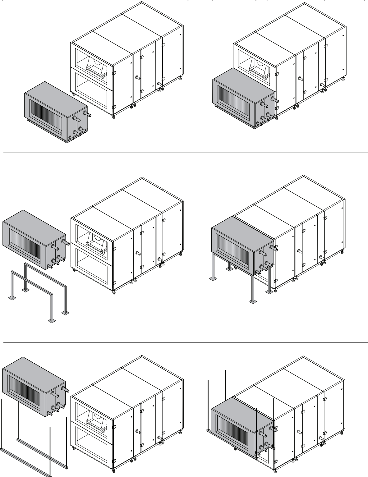
Rys. 17. Przykłady montażu sekcji nagrzewnicy/chłodnicy
