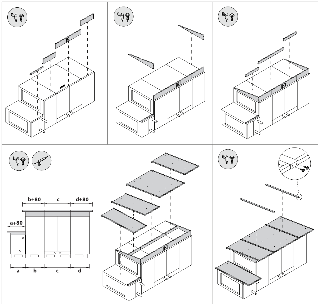
Rys. 27. Montaż osobno zamawianego dachu ochronnego 1
